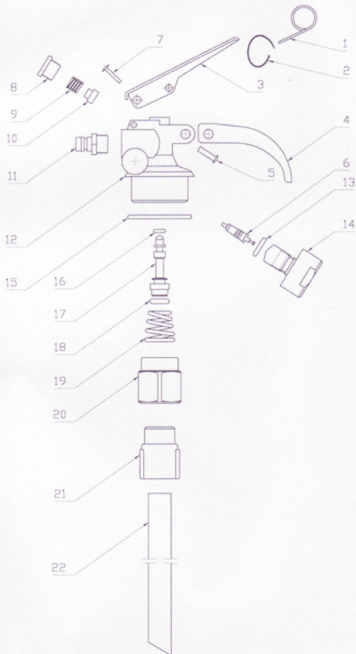
Zawór do gaśnicy GP-2X
